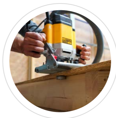
Roulement à débords Pour débords de panneaux jusqu'à 15 mm
